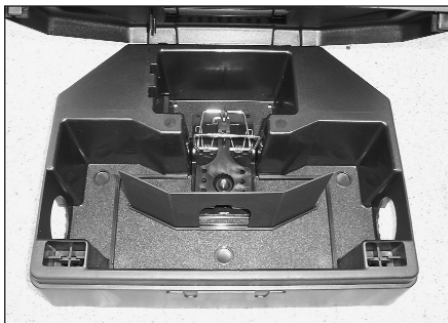
Ratière Big Snap-E illustrée dans la station modulaire d'appât AEGIS MC .
